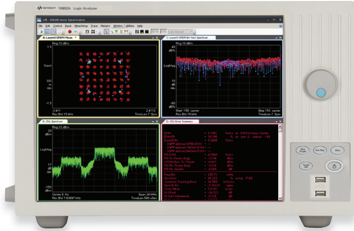
그림 4. 로직 분석기에서 실행되는 키사이트의 89600 벡터 신호 분석 소프트웨어를 이용해서 디지털 베이스밴드와 IF 신호에 대해 심층적인 시간, 주파수, 변조 도메인 분석을 수행
