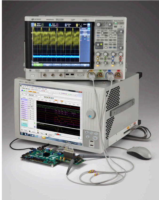
그림 3. 뷰 스코프 (View Scope)는 스코프와 로직 분석기 파형을 단일 디스플레이에 원활하게 통합
