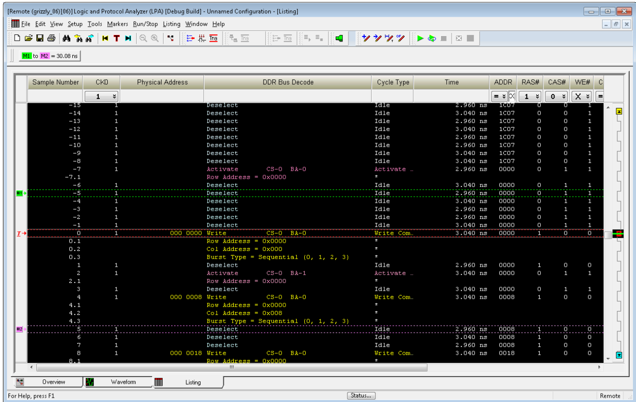
16850 시리즈 캡처 및 DDR3 Addr/Cmd 라인 디코딩
