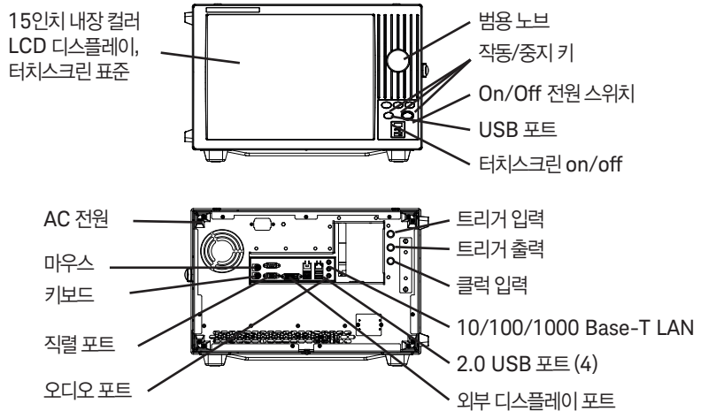
그림 10. 16850시리즈 전면판 및 후면판
