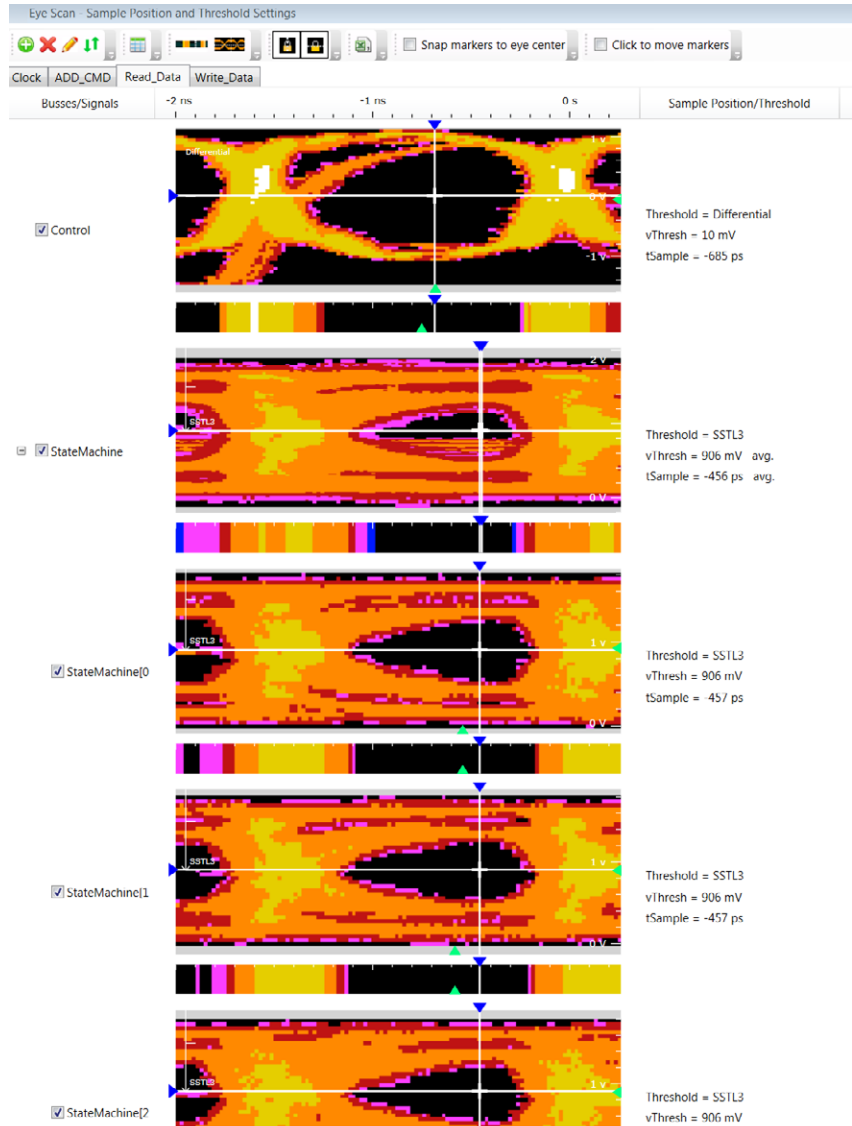
그림 2. 아이(eye) 스캔은 정확한 스테이트 캡처를 위한 샘플 위치를 자동으로 설정하며, 추가 오실로스코프 없이 각 입력 신호에 대한 신호 무결성 보기를 제공
